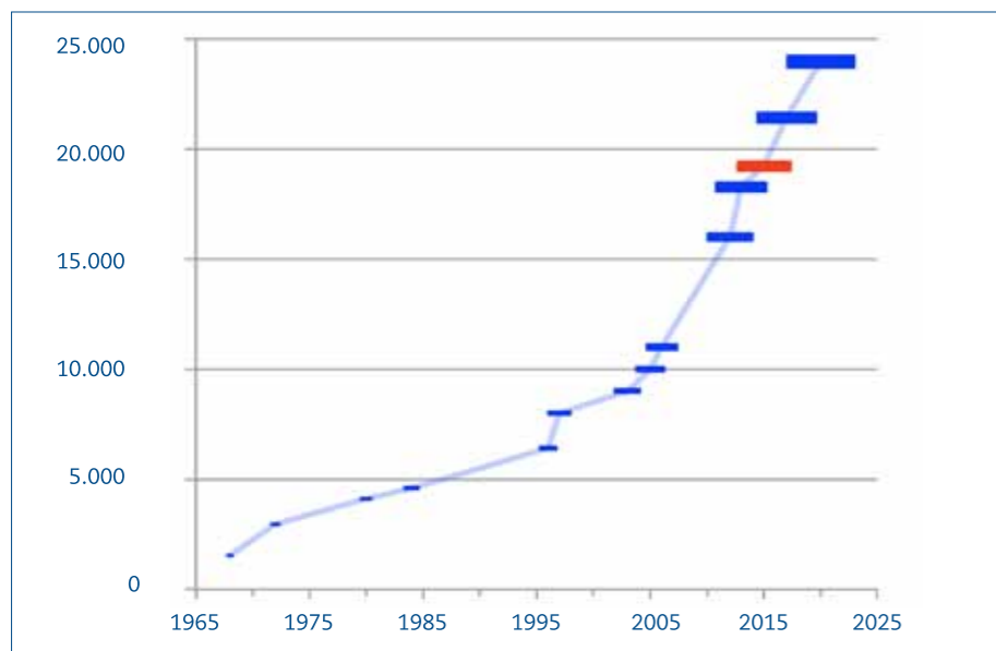
Entwicklung der Tragfähigkeit von Containerschiffen von 1968 bis 2020 in TEU [Standardcontainer], rot markiert die Größe der 2015 gebauten „MSC Zoe“.
